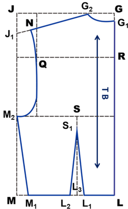
Gambar 2.10 Pola Dasar Badan Belakang dengan Sistem Praktis
