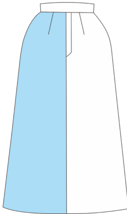
Gambar 2.17 Contoh Pola Dasar Rok Bagian Belakang
